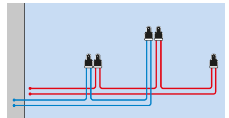
Ringleitung
